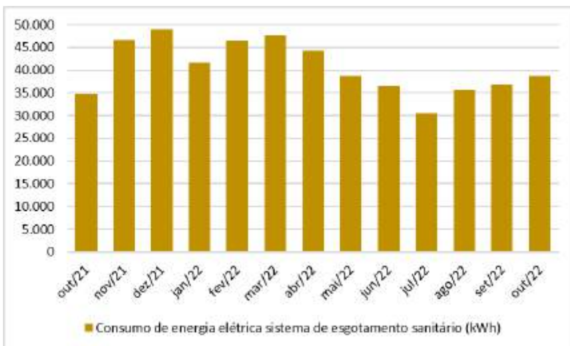
Figura 7-9: Consumo de energia elétrica – Cesan
