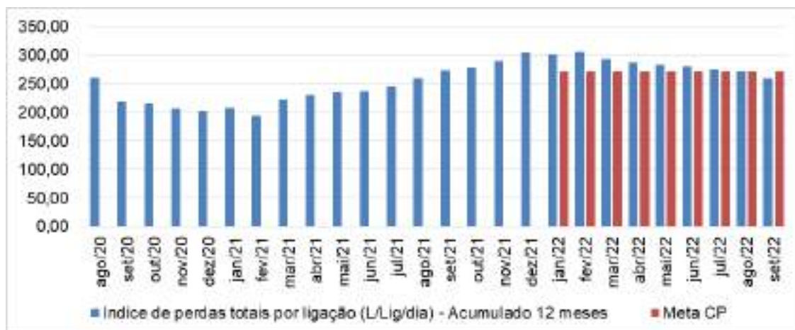
Figura 6-29: Índice de perdas por ligação - Cesan
