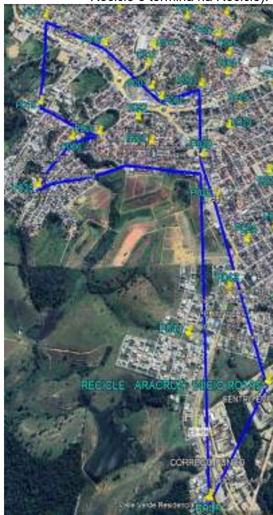
Figura 35-29: Sequência dos pontos a serem atendidos pelo veículo 2, viagem 2 (viagem inicia na Recicle e termina na Recicle).
