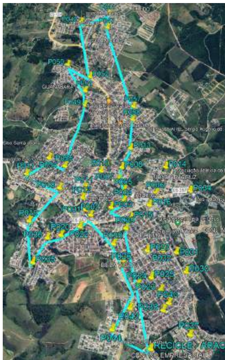
Figura 35-13: Sequência dos pontos a serem atendidos pelo veículo 1, viagem 2 (viagem inicia e termina na Recicle).
