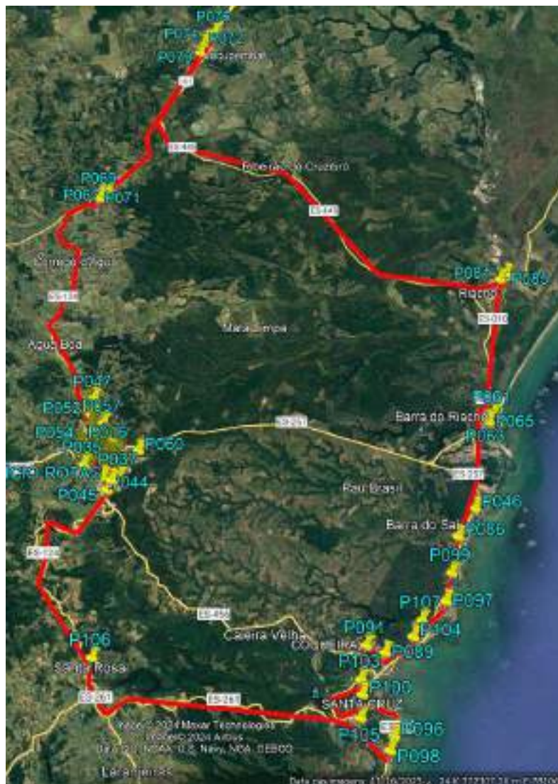
Figura 35-6: Sequência dos pontos a serem atendidos pelo Veículo 3 (viagem inicia e termina na Recicle), somente segundas, quartas e sextas-feiras.
