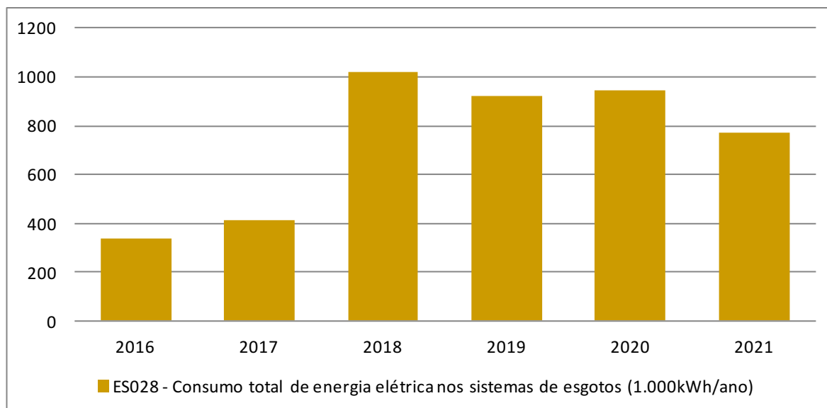
Figura 7-8: Consumo de energia elétrica dos sistemas de esgotamento sanitário – SAAE
