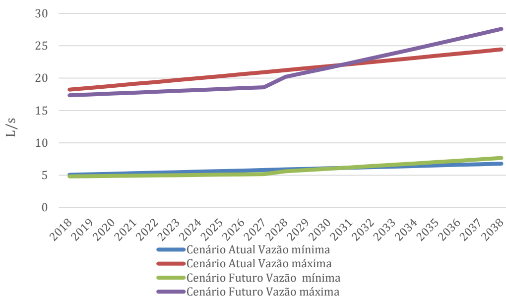
Figura 16 – Vazões estimadas – cenário atual e futuro
